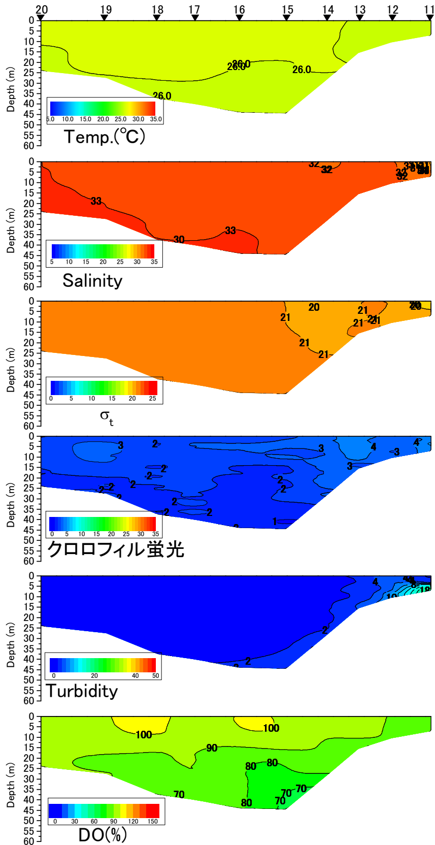
八代海中央ラインの水温(°C)、塩分、密度( \sigma_t )、クロロフィル蛍光強度、濁度、溶存酸素飽和度(DO%)の鉛直面図(国土交通省の調査による) (2016年9月2日)
